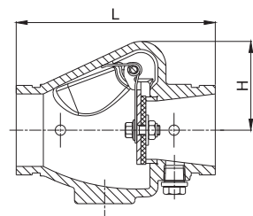
FIG. FFA-F3322B
