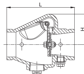
FIG. FFA-F3322
