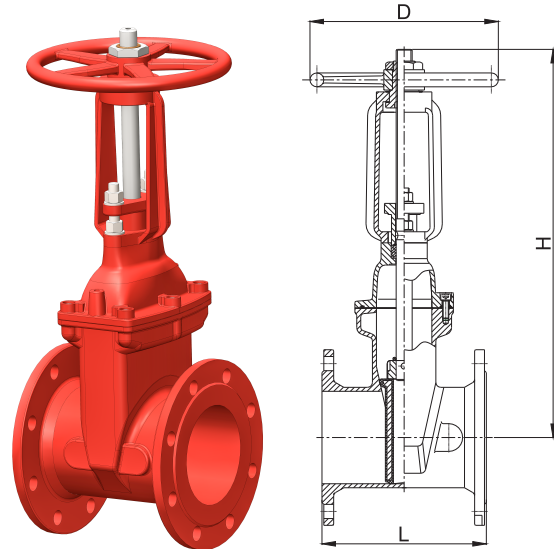
FIG. FFA-F0199-F, FL X FL Ends
